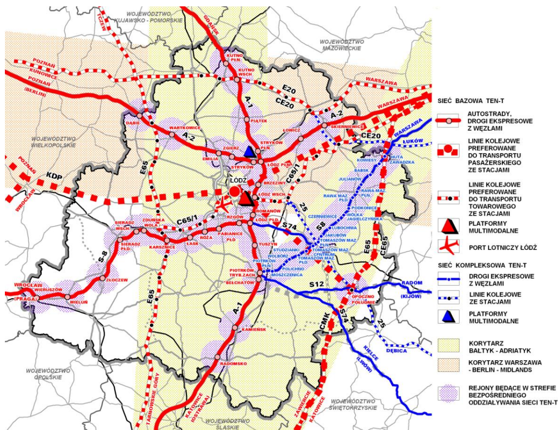
Rys. 135. Obszary Strategicznej Interwencji wynikające z polityki rozwoju województwa łódzkiego – rejonory będące w strefie bezpośredniego oddziaływania sieci TEN-T
